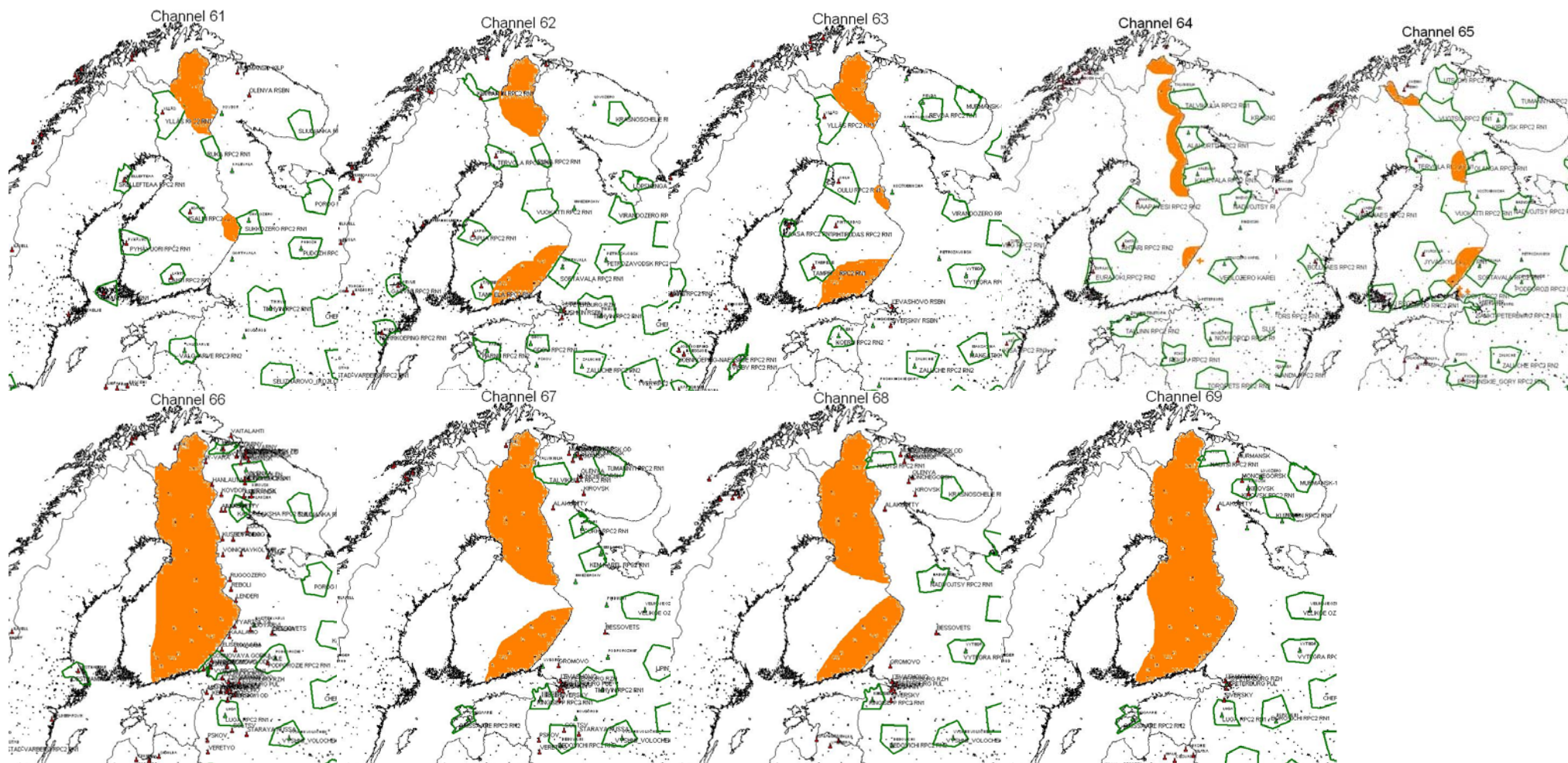
Kanavakohtainen suuntaa antava arvio pääasiassa Venäjän taajuuksienkäytön aiheuttamista rajoitteista (värjätyt alueet) matkaviestintukiasemille (790-862 MHz).
