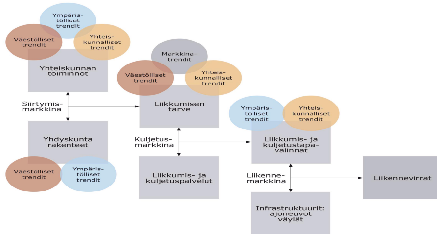
Kaavio 3. Eri tekijöiden vaikutukset liikennevirtojen syntymiseen
