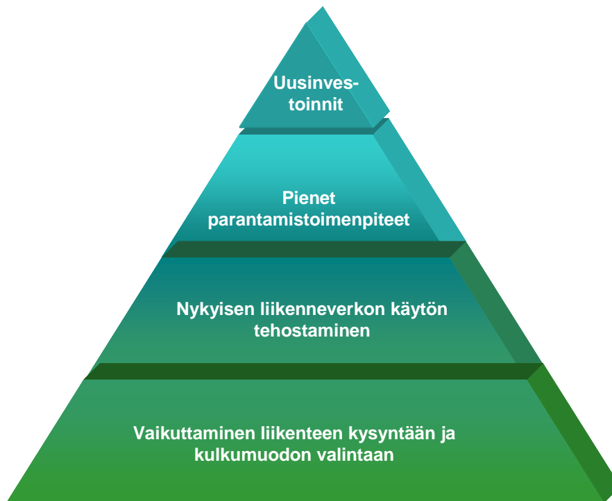
Kuva 1 Liikennejärjestelmän neliporrasperiaate
